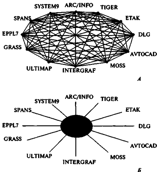
Рис. 52. Преимущества разработки и поддержки N -программными средствами единого обменного формата (SDTS): количество необходимых конвертеров уменьшается с N(N-1) в случае A до 2N в случае B
